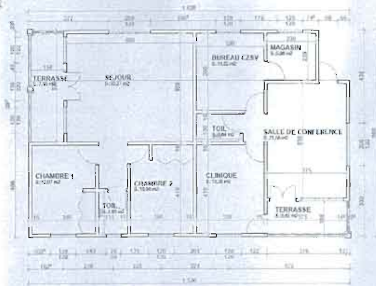
PLAN DE DISTRIBUTION
