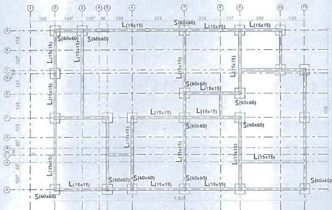
PLAN DE FONDATION
